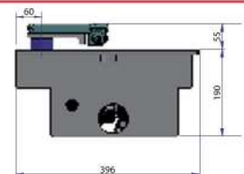
Particular de la centralita y gato
